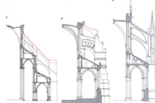
飞扶壁 Flying Buttresses (红色部分)
