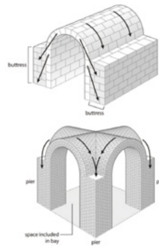
罗马筒形拱和拱券空间示意
